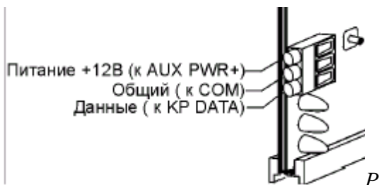
ИС. 2. ПОДКЛЮЧЕНИЕ ПРИЕМНОГО МОДУЛЯ.
