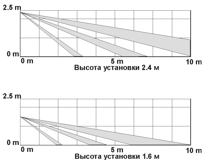
Рис. 3. ДИАГРАММА ЗОНЫ ОБНАРУЖЕНИЯ. ВИД СБОКУ.
