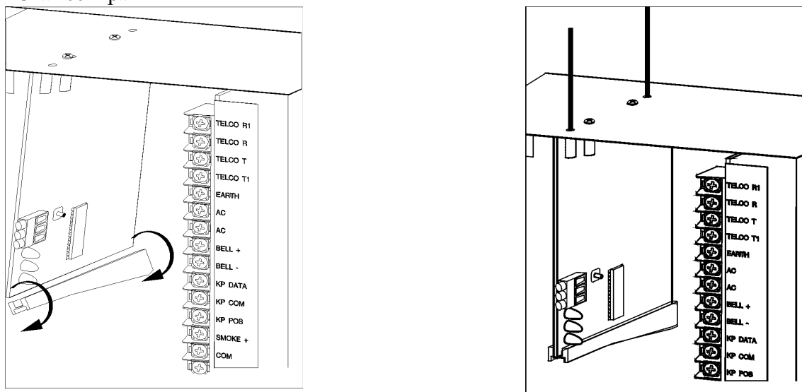
Рис. 1. УСТАНОВКА ПЛАТЫ ПРИЕМНИКА В КОРПУС БАЗОВОГО БЛОКА.
