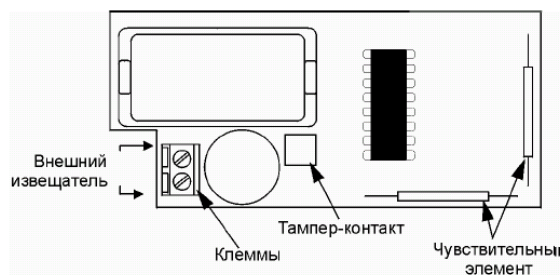
Рис.3. Вид ИЗВЕЩАТЕЛЯ С О СНЯТОЙ КРЫШКОЙ.
